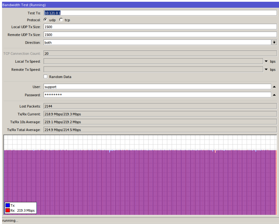
Рис.3 РТР650 12 км, 45 МГц, 215+215 =430 Mbps Duplex UDP 1500 bytes
