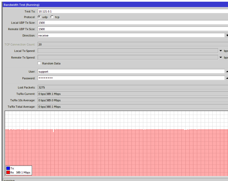
Рис.2 PTP650 12 км, 45 MHz, 390 Mbps Download UDP 1500 bytes
